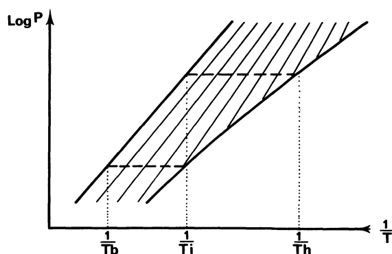
Fig. 4. — Diagramme pression température et cycle thermochemique SL-G.
