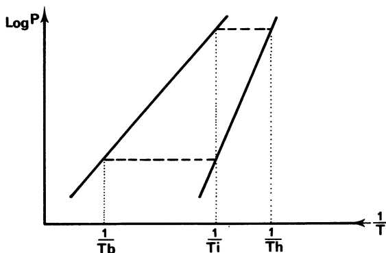
Fig. 2. — Diagramme pression-température et cycle thermo-chimique SS-G.
